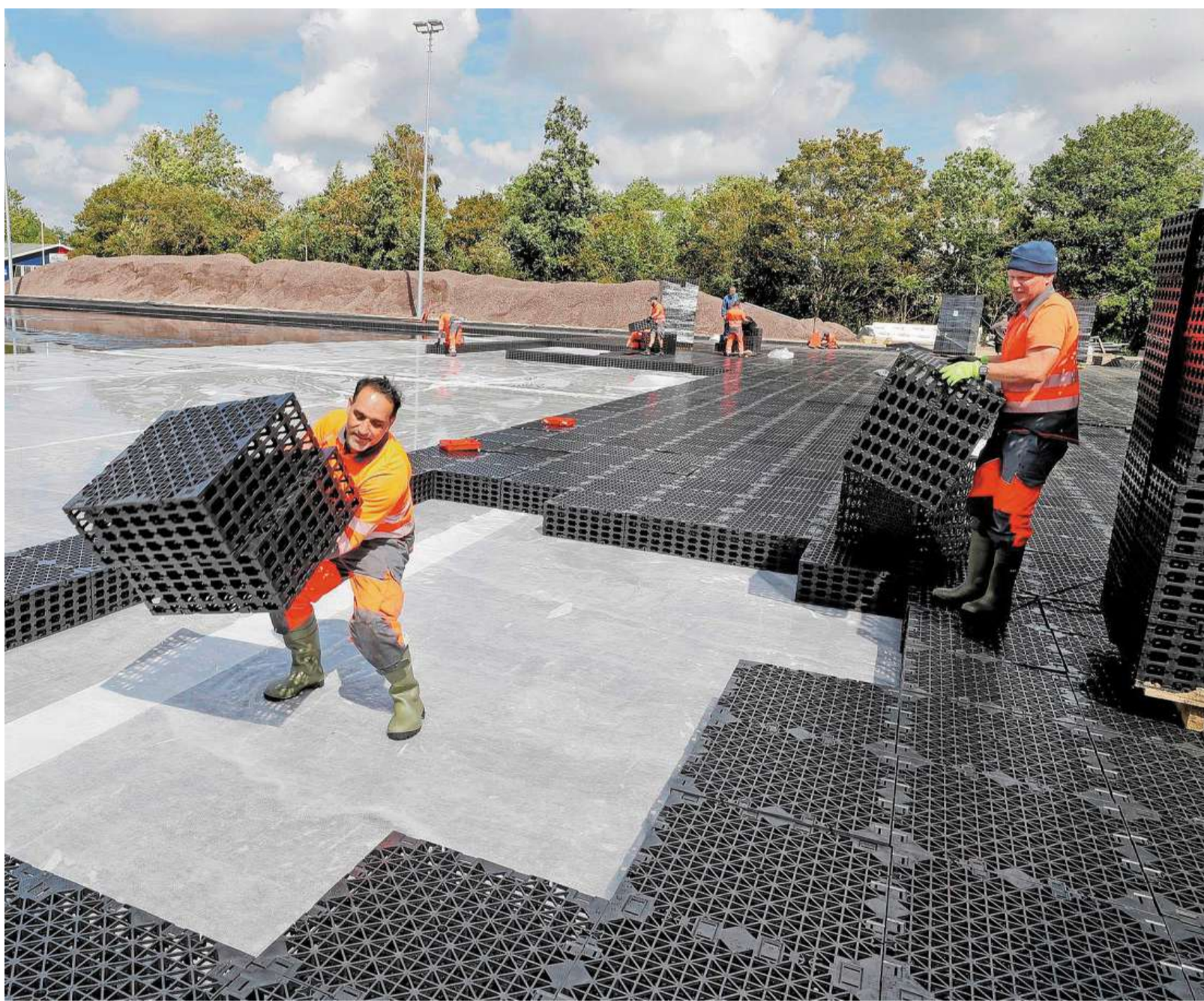
Op het terrein van hockeyvereniging Magnus in Schagen wordt het waterveld aangelegd. De kratjes gaan de waterberging vormen.
